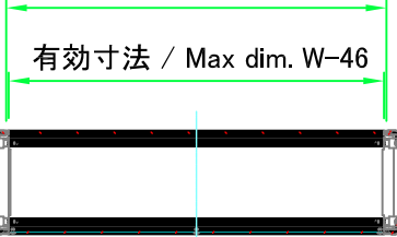
ハメ込みパネル有効寸法 / Slide panel Max dim. W-40
