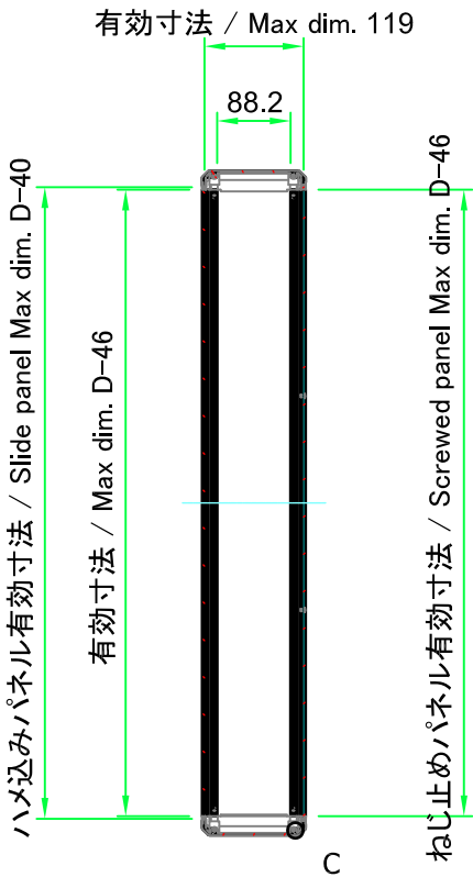
B-B ( 1 : 10 )
